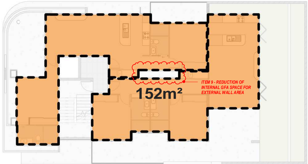
Plan LEVEL 1 - GFA 1 : 150
