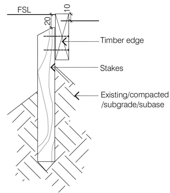
6 EDGE TYPE 2 - TIMBER EDGE
