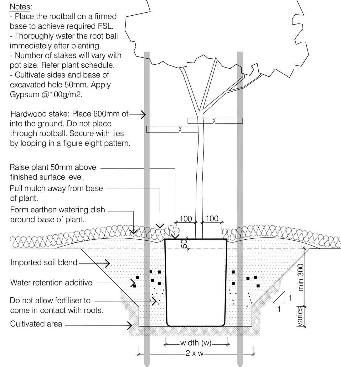
3 PLANTING DETAIL: 45-200Ltr
